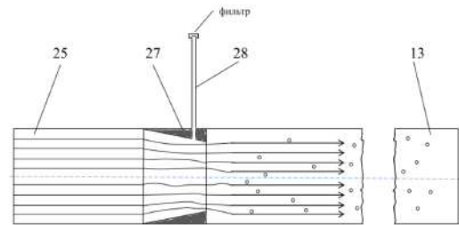
Рис. 4. Конструктивная схема водовоздушного эжектора
