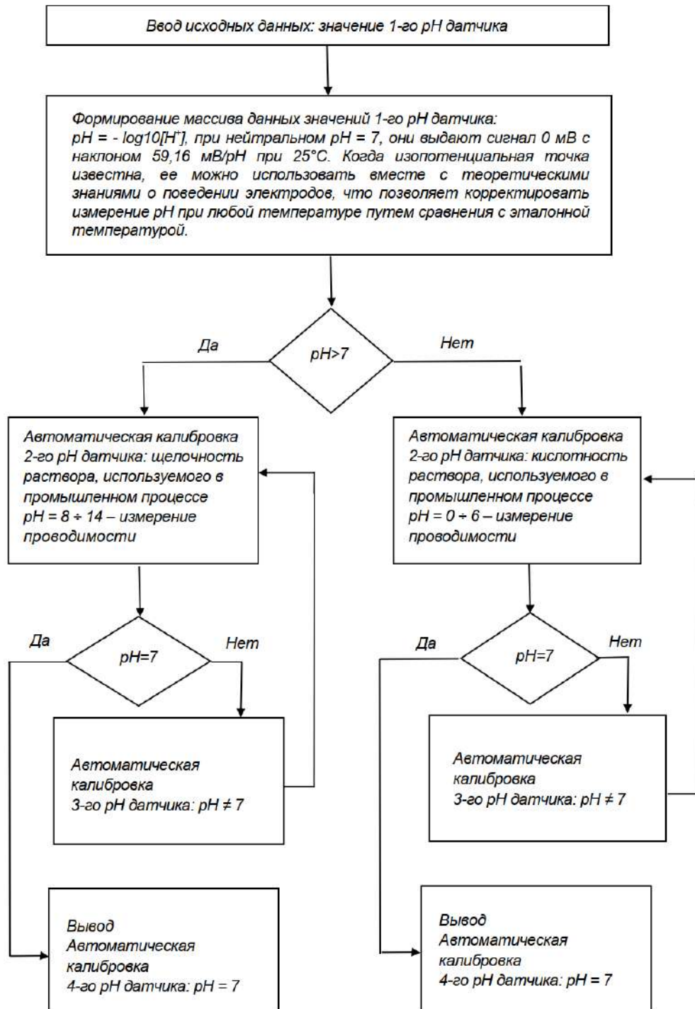
Рис. 6. Блок-схема алгоритма работы модуля управления установкой
