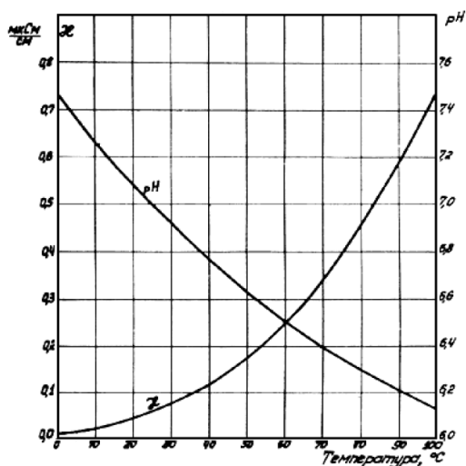
Рис. 1. Влияния температуры на электрическую проводимость и степень кислотности (pH) чистой воды
