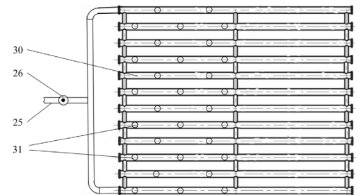
Рис. 5. Схема компоновки трубок успокоительной решетки (распределительного коллектора)
