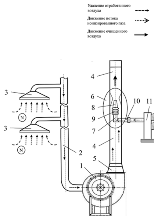
Рис. 1. Принципиальная конструктивно-технологическая схема системы
