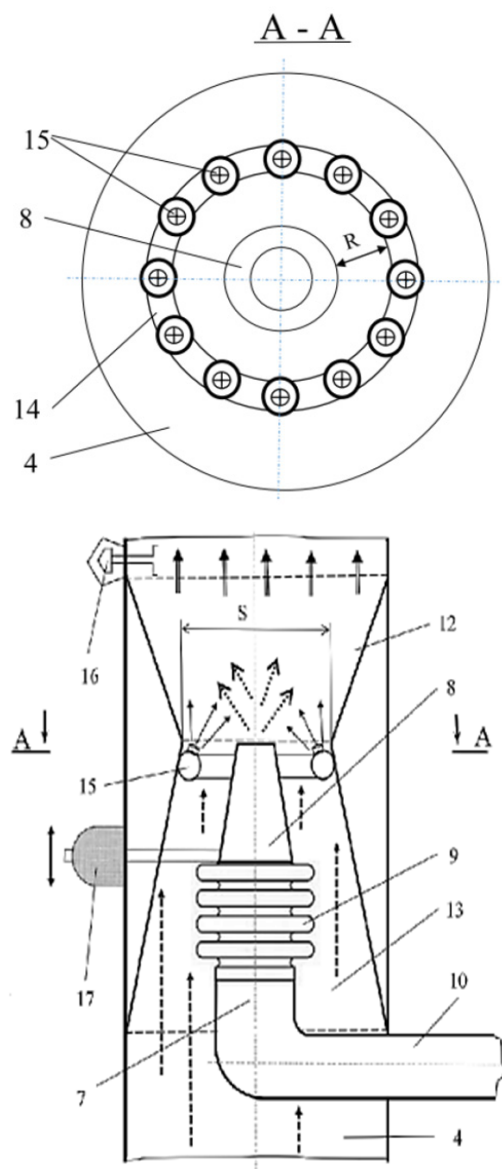
Рис. 2. Принципиальная схема модуля смешивания
